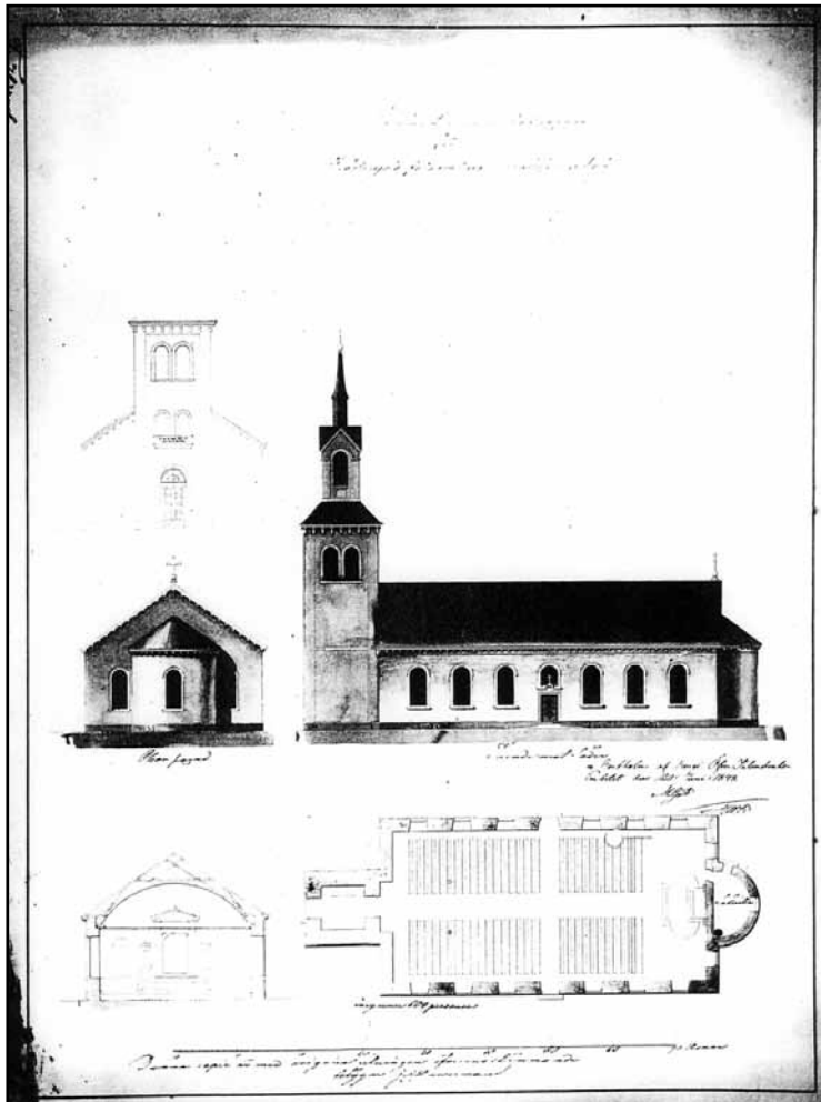
Arkitekt Johan Adolf Hawermans ritning till ny kyrka i Fröderyd från 1848. ATA.
