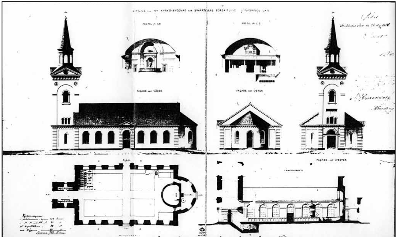
Arkitekt Ludvig Hedins slutliga ritning till ny kyrka för Svarttorp. ATA.
