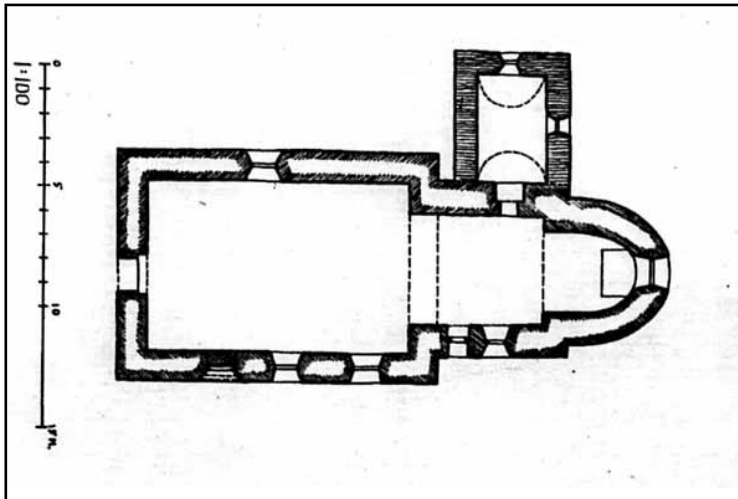
Uppmätning av Myresjö ödekyrka, utförd av Sven Brandel 1925. ATA.
