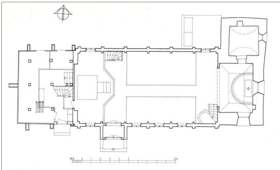
Plan över Haurida kyrka upprättad av G Wirén 1980. Ritning från Ullén, 1983.
