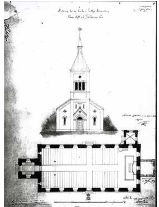
Hultsjö kyrka, enligt förslag från Axel Nyström. Historiserande dekorationer på fasaden togs bort när kyrkan väl uppfördes. I det slutliga ritningsförslaget ändrades också placeringen av sakristian - den först föreslagna placeringen norr om koret finns här kvar jämsides med aktuell justering. Ritning från ATA.
