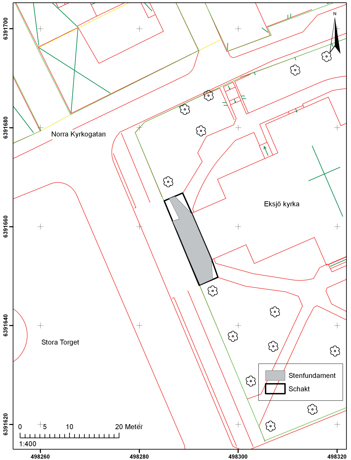
Schaktet och det påträffade stenfundamentet, markerat i grått, utanför Eksjö kyrka.
